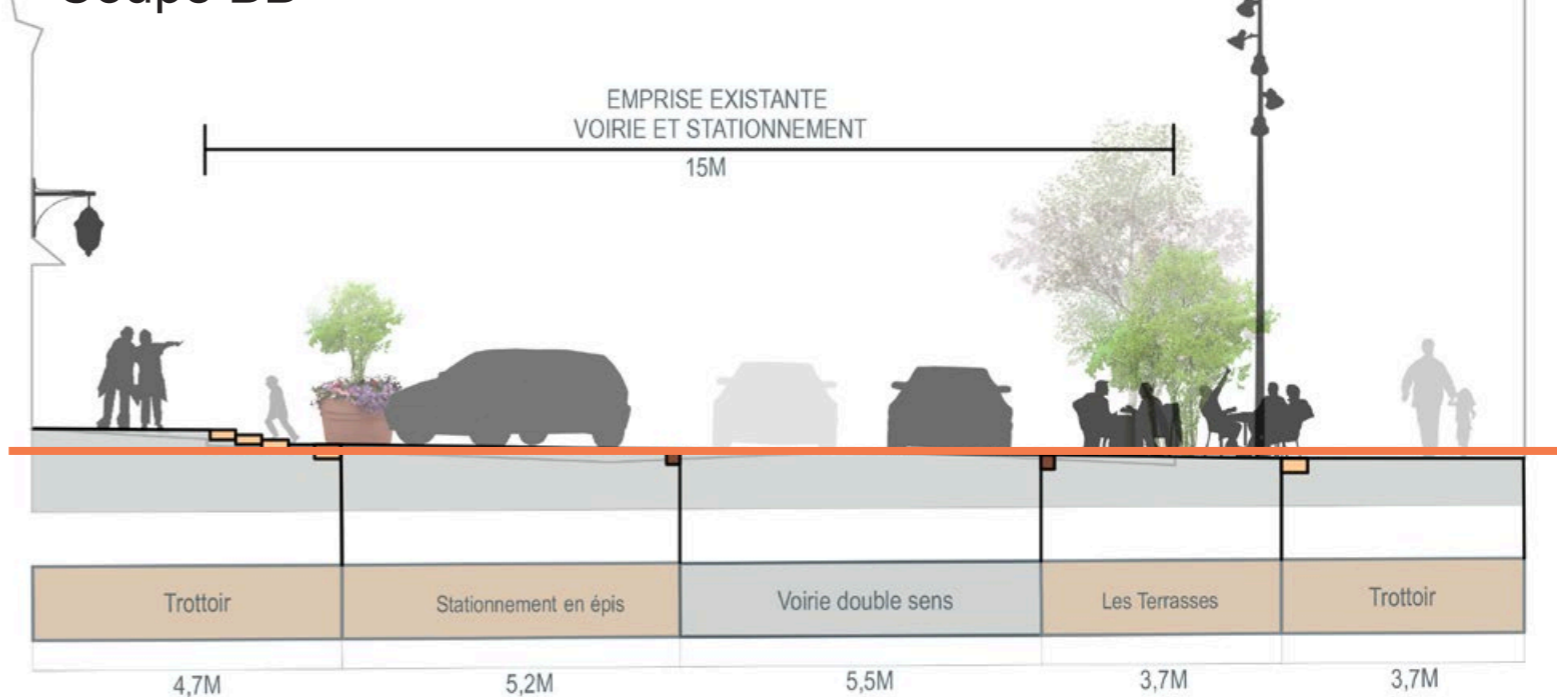
Coupe BB'
