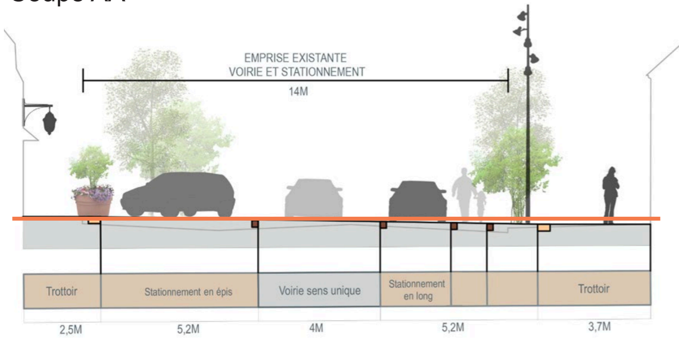
Coupe AA'
